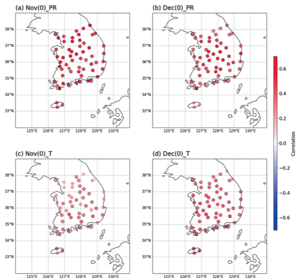
그림 9.2 Nino3 지수와 한반도 11월, 12월 온도, 강수와의 상관관계(1980~2023년). 90% 유의수준에서 유의미한 관련성은 닫힌원으로 표시.
