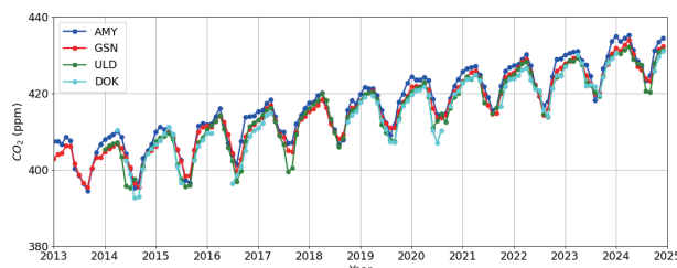
그림 2.1 2013~2024년의 기간 동안 안면도(AMY), 고산(GSN), 울릉도(ULD), 독도(DOK)의 이산화탄소 배경농도(국립기상과학원, 2025).
