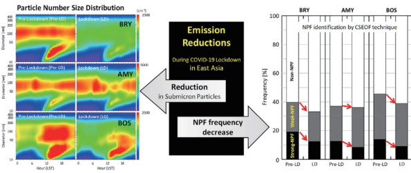
그림 6.2 COVID-19 기간 한반도 배경대기지역(백령도, 안면도, 제주도)에서 관측된 입자생성 및 성장 현상의 감소(Park et al., 2023).
